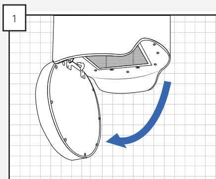
1 Öppna luckan genom att dra nedåt i luckans kant framtill på fläktkåpan.
