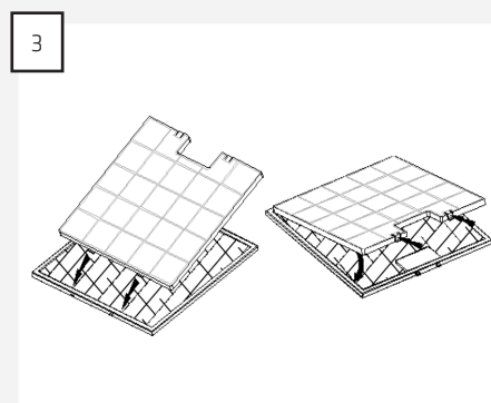
3 Monter recirkulationsfilteret bag på stålfilteret.
